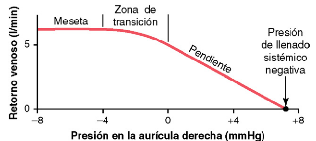
Figura 20-9 Curva de retorno venoso normal. La meseta está provocada por el colapso de las grandes venas que entran en el tórax cuando la presión en la aurícula derecha desciende por debajo de la presión atmosférica. Obsérvese también que el retorno venoso se vuelve a cero cuando la presión en la aurícula derecha aumenta hasta una presión media igual a la del llenado sistémico.
